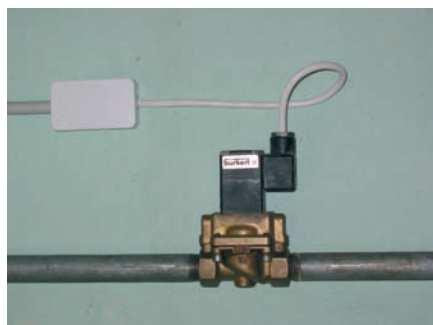
Magnetventil
